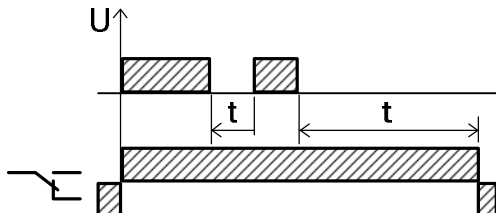
Диаграмма работы 31
