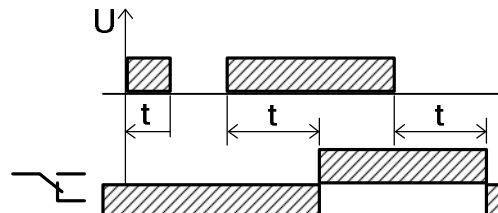
Диаграмма работы 31
