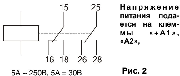
Схема подключения
